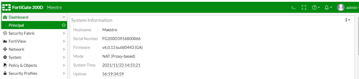
Ilustración 227 – Firewall
