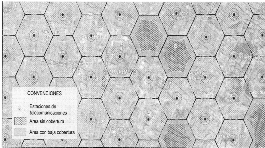
Ilustración 2. Cobertura red móvil
