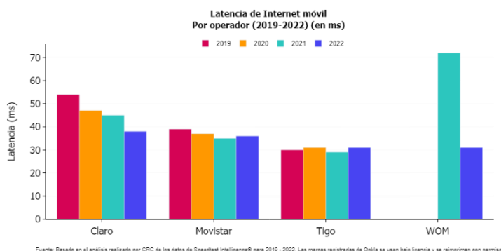
Gráfico 34. Indicadores latencia de calidad de Internet Móvil en “Mediciones de calidad desde la experiencia del usuario”, 20-9 - 2022.
